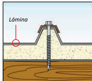
Perfil fijar a Madera HY01
