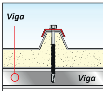
Perfil fijar a Metal AB01
