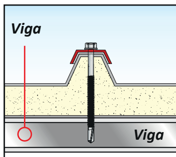
Perfil fijar a Metal TX01
