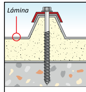
Perfil fijar a Concreto GZ01
